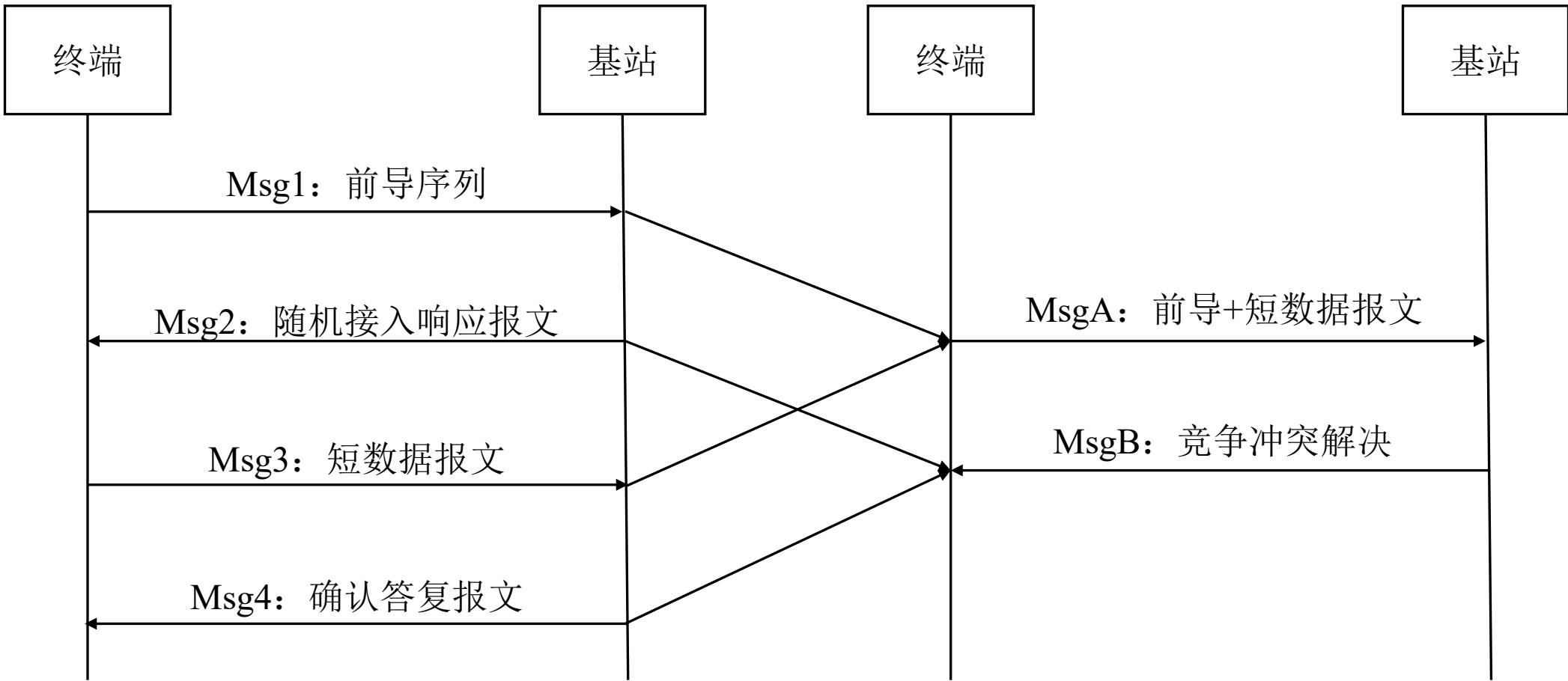
四步SDT 随机接入过程
